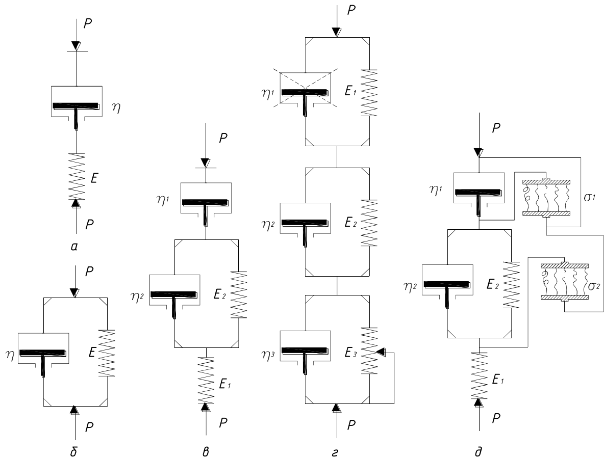
Рисунок 1 – Схеми реологічних моделей (використовуються до опису процесу стискання): а-«тіло Максвелла»; б-«тіло Кельвіна» (модель Кельвіна-Фойгта-Мейєра); в-чотирипараметрична модель волокнистого високополімерного матеріалу (Алфрея); г-трихланкова модель Кукіна-Соловйова; д-модель Алфрея з доданими елементами руйнування
